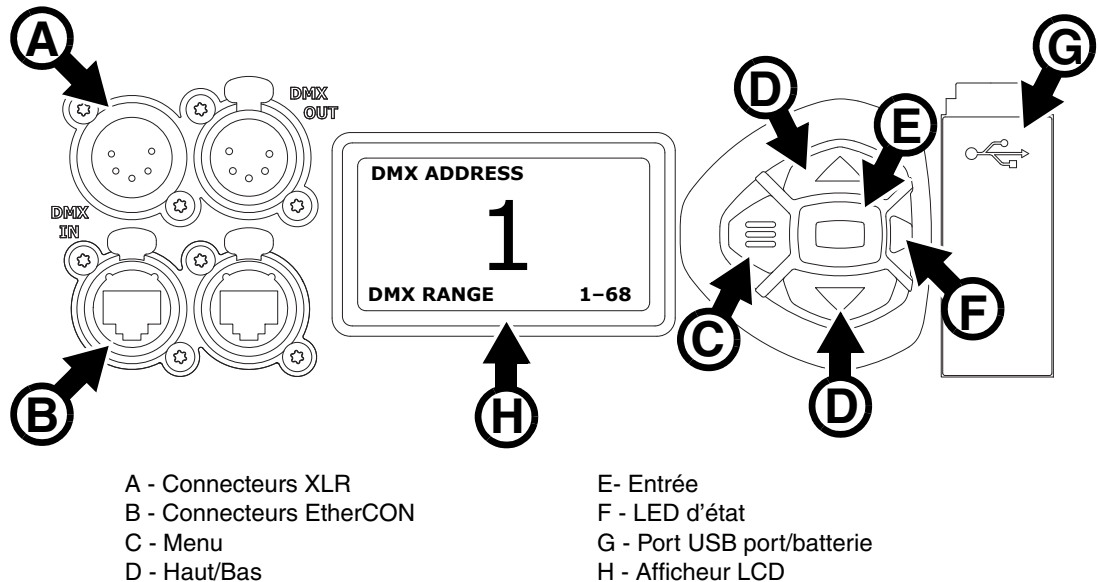
Figure 3 : Afficheur et panneau de contrôle
