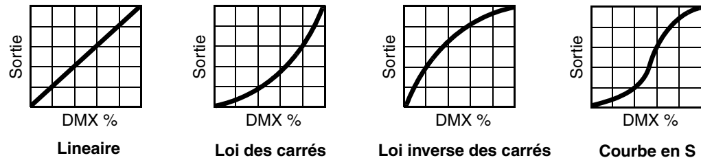
Figure 4 : Courbes de gradation
