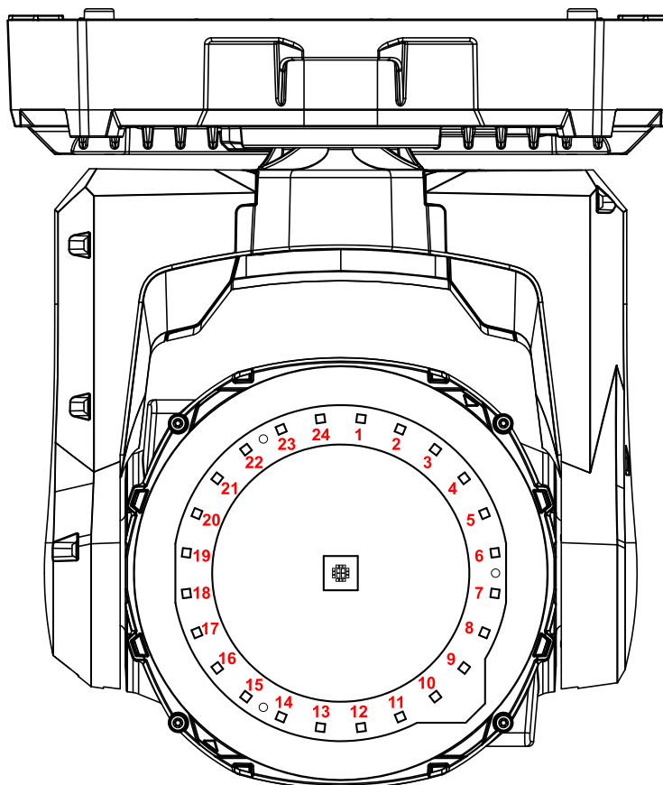
MAC One Backlight Pixelanordnung
